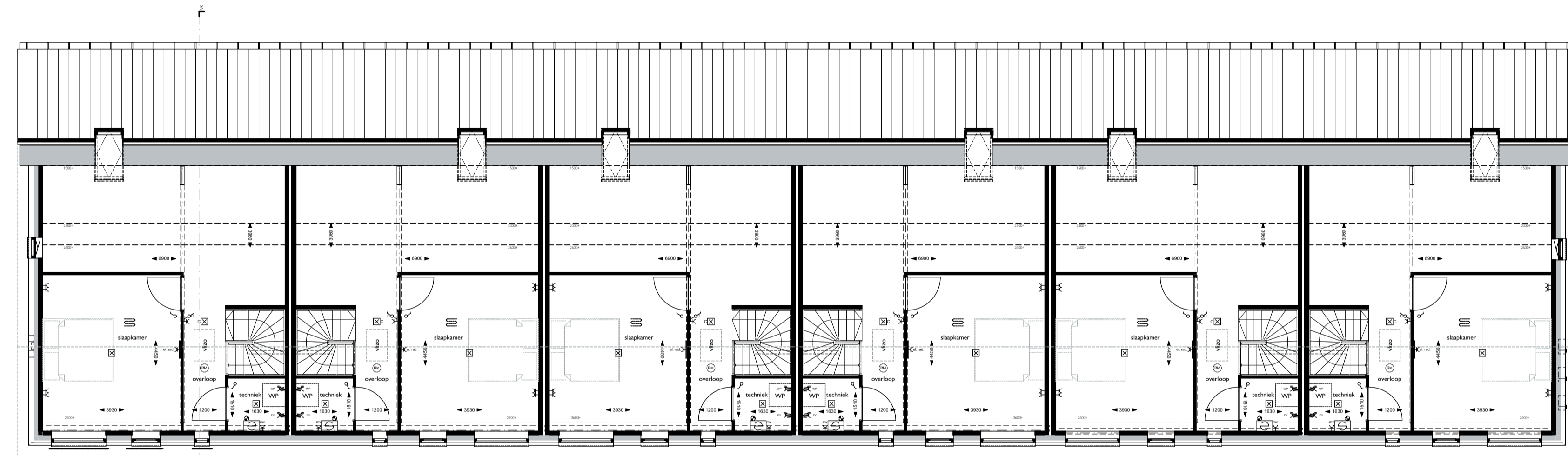
1e verdieping
