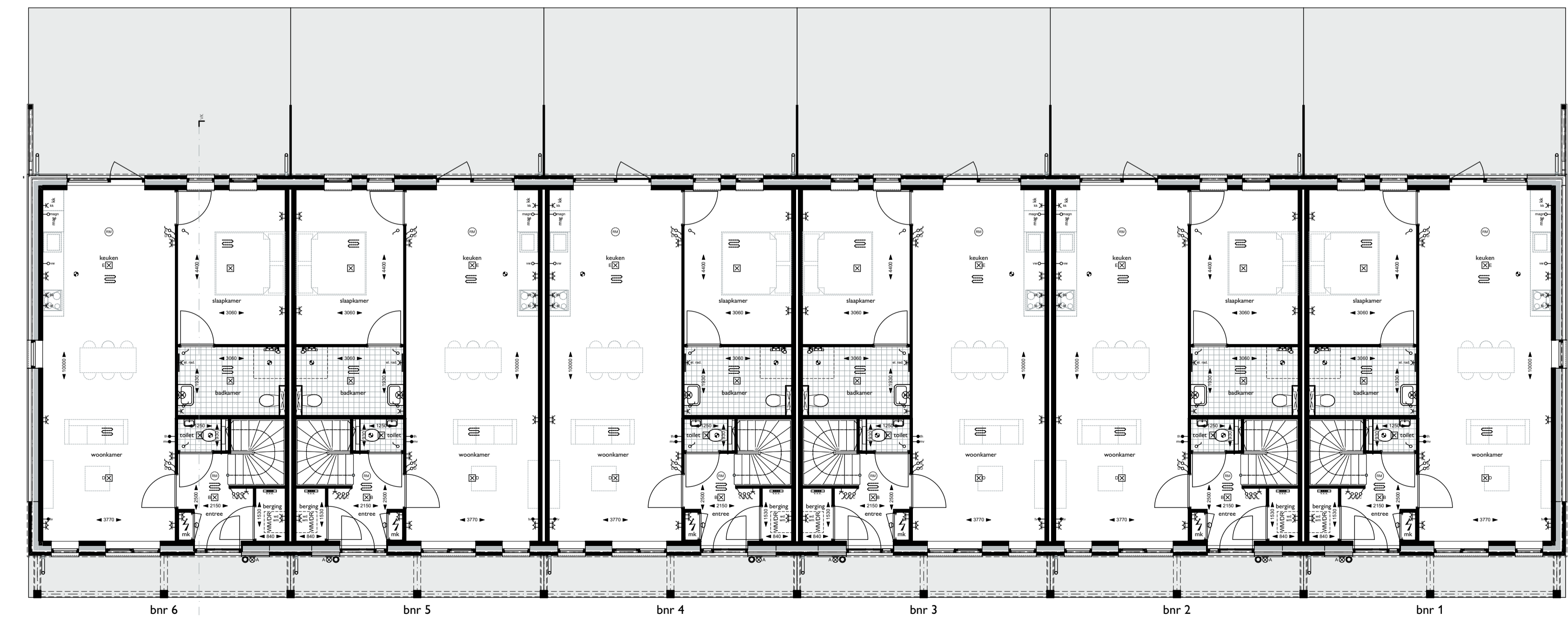
Begane grond
