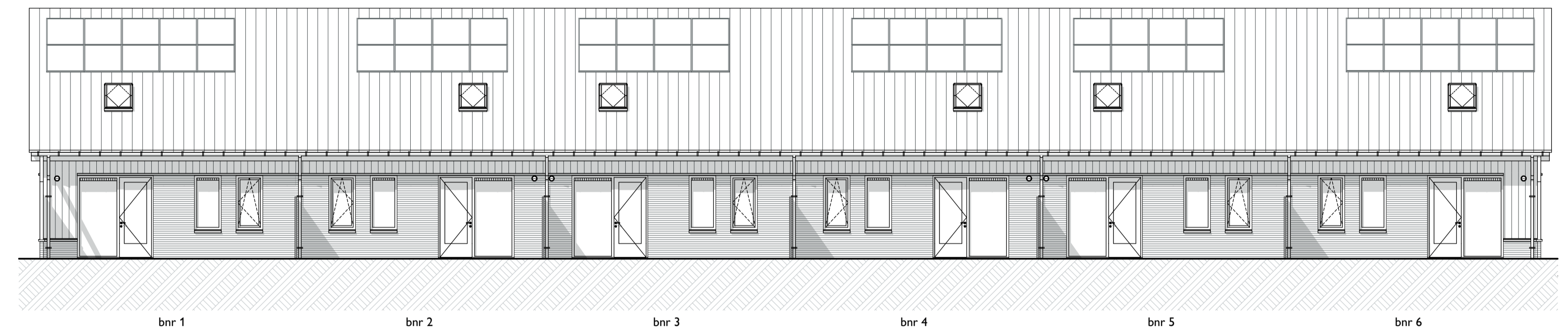
Achtergevel
