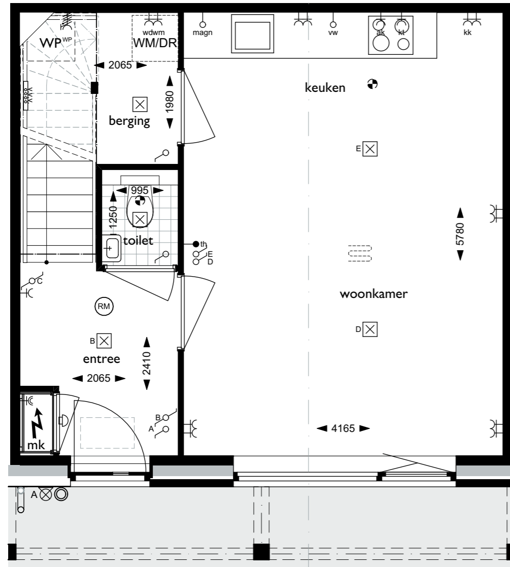
Begane grond
