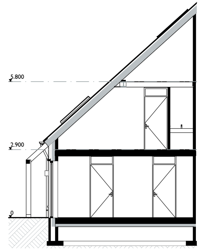
Doorsnede VK-VK
