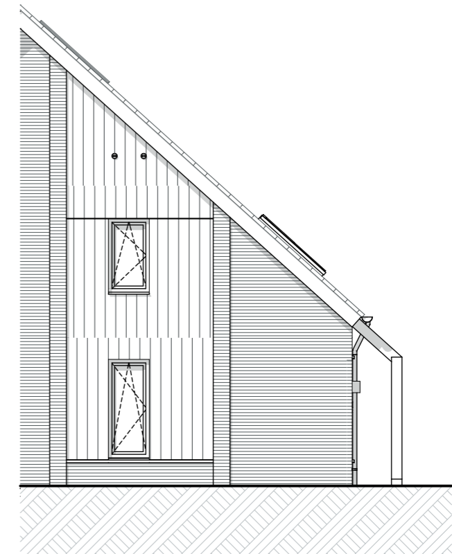
Linkergevel
