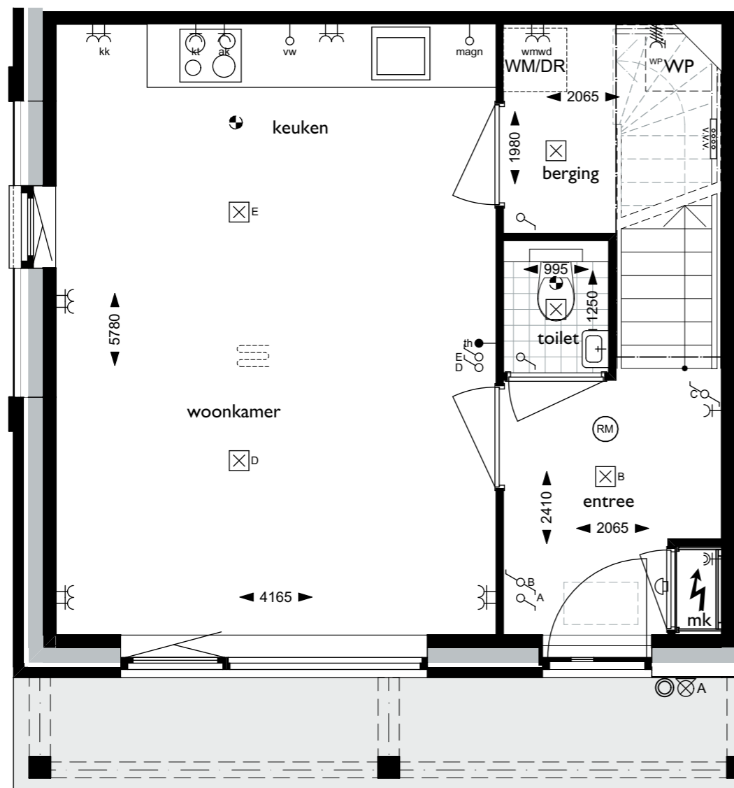
Begane grond
