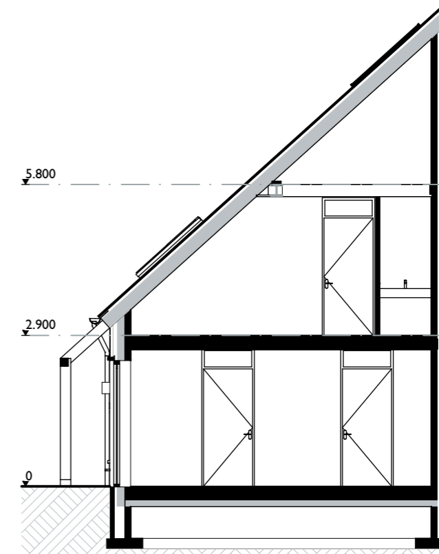
Doorsnede VK-VK
