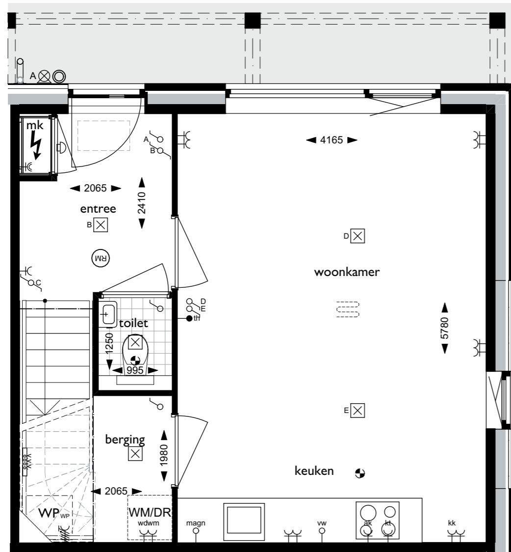
Begane grond
