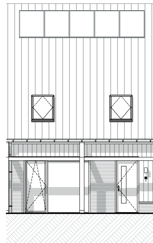
Voorgevel
