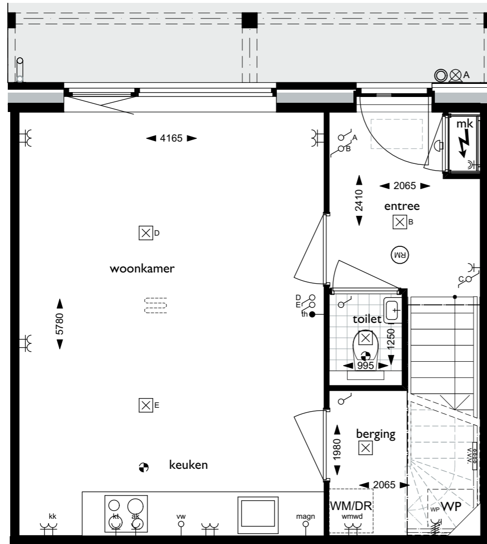
Begane grond
