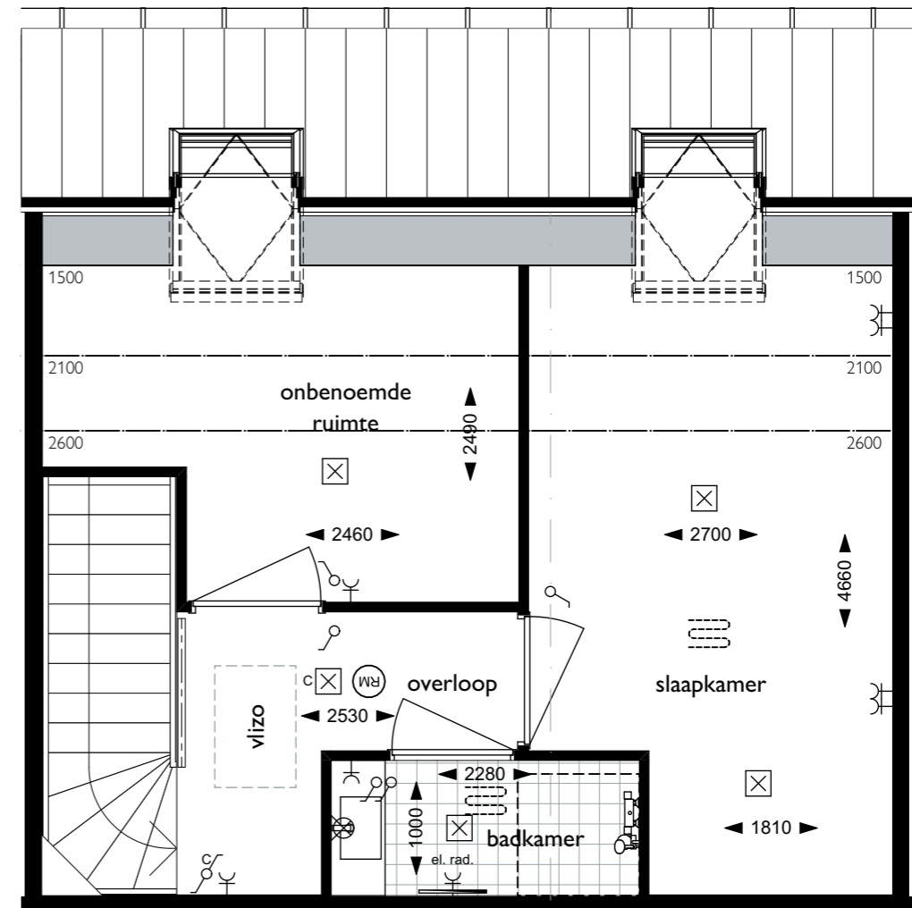
1e verdieping
