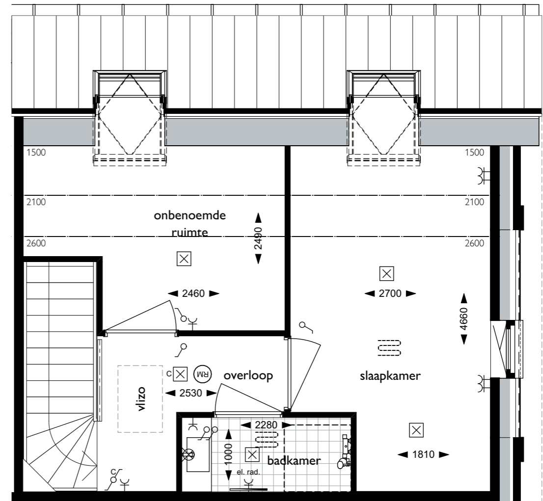
1e verdieping
