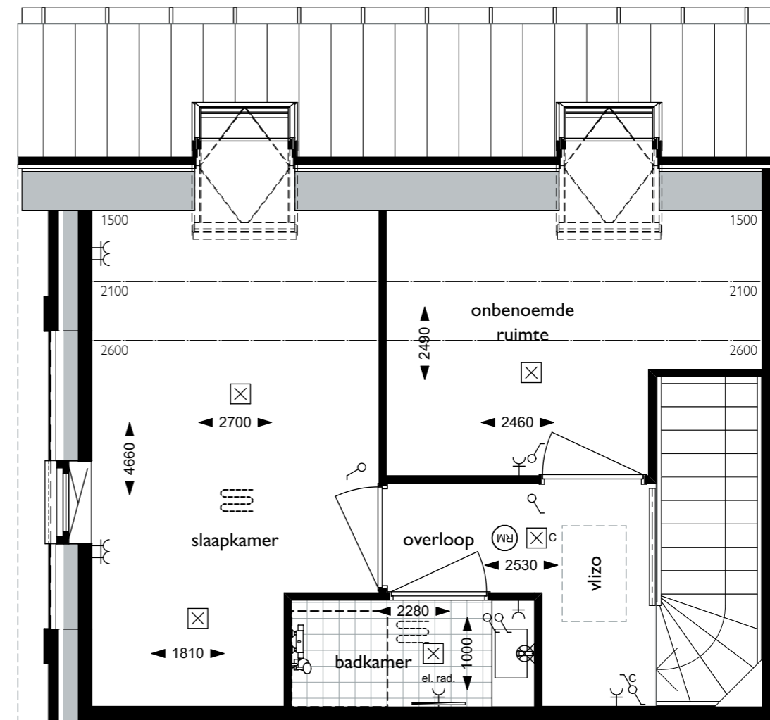
1e verdieping
