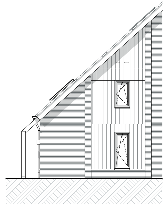
Rechtergevel
