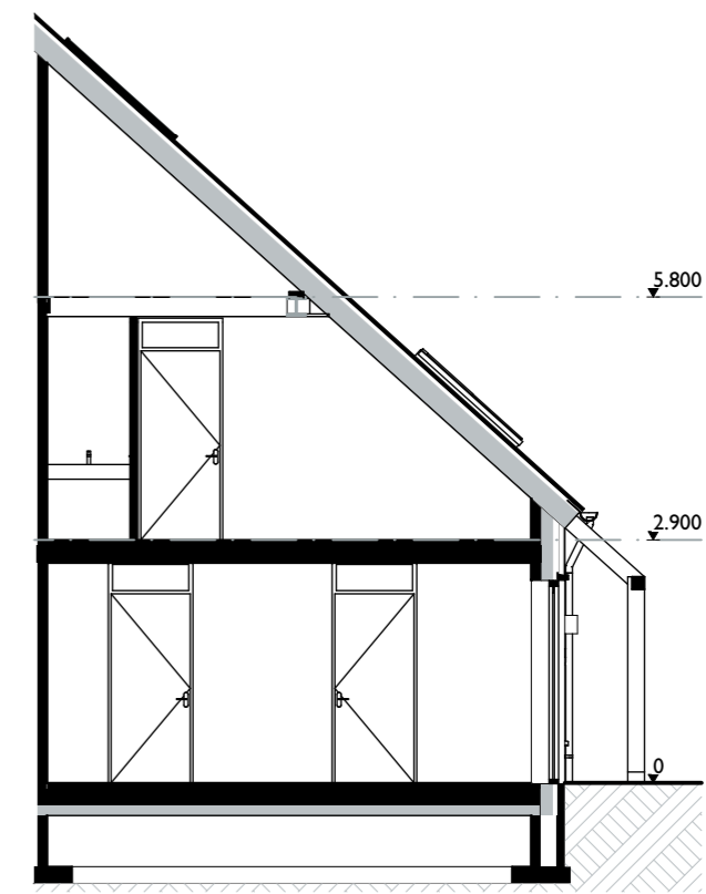
Doorsnede VK-VK
