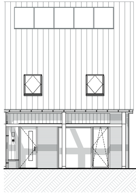
Voorgevel
