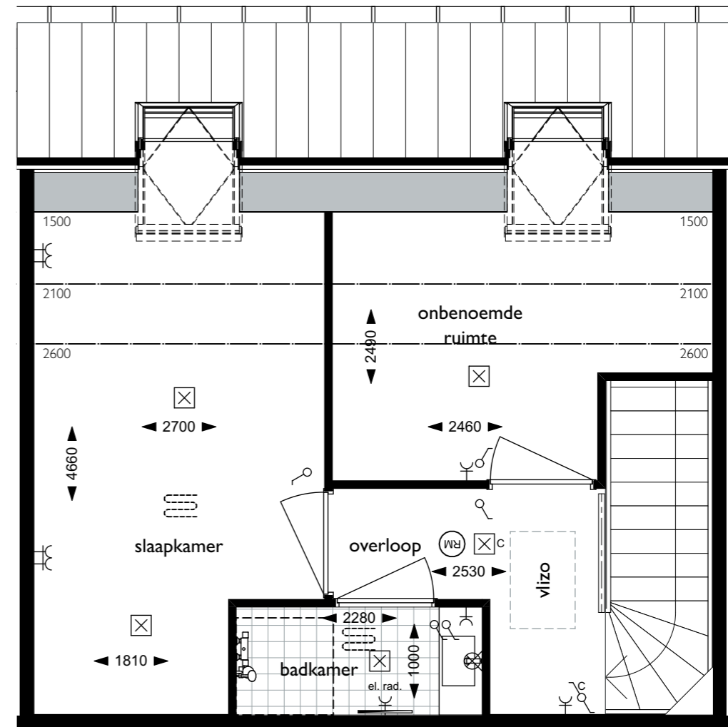
1e verdieping
