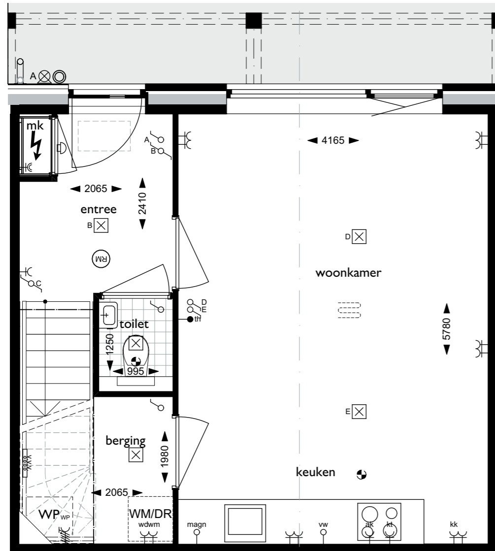
Begane grond
