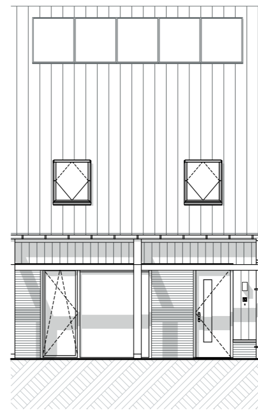
Achtergevel
