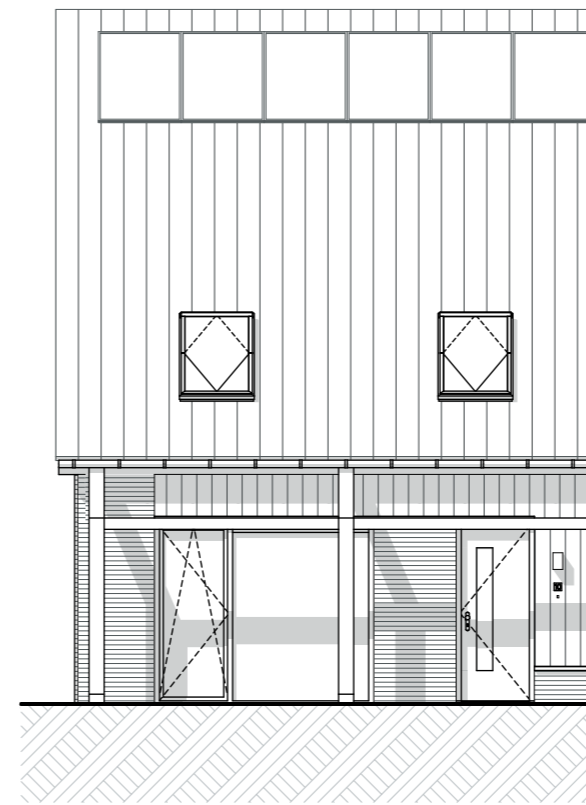
Voorgevel
