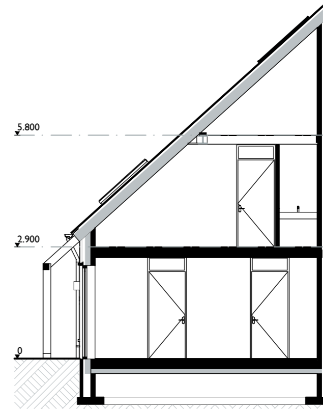
Doorsnede VK-VK
