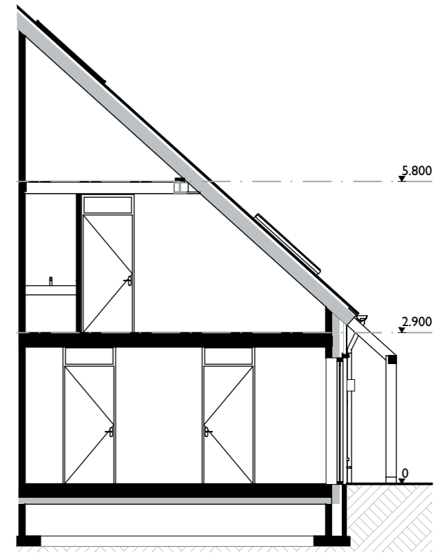
Doorsnede VK-VK
