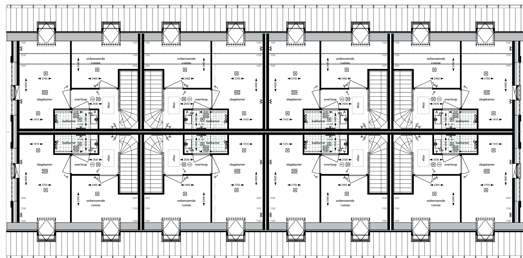
1e verdieping
