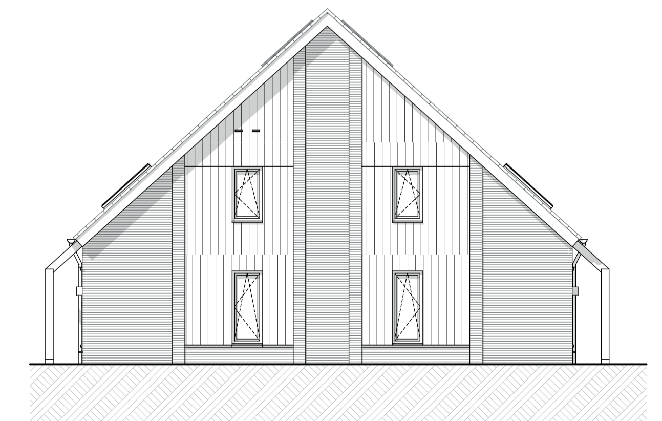
Rechtergevel
