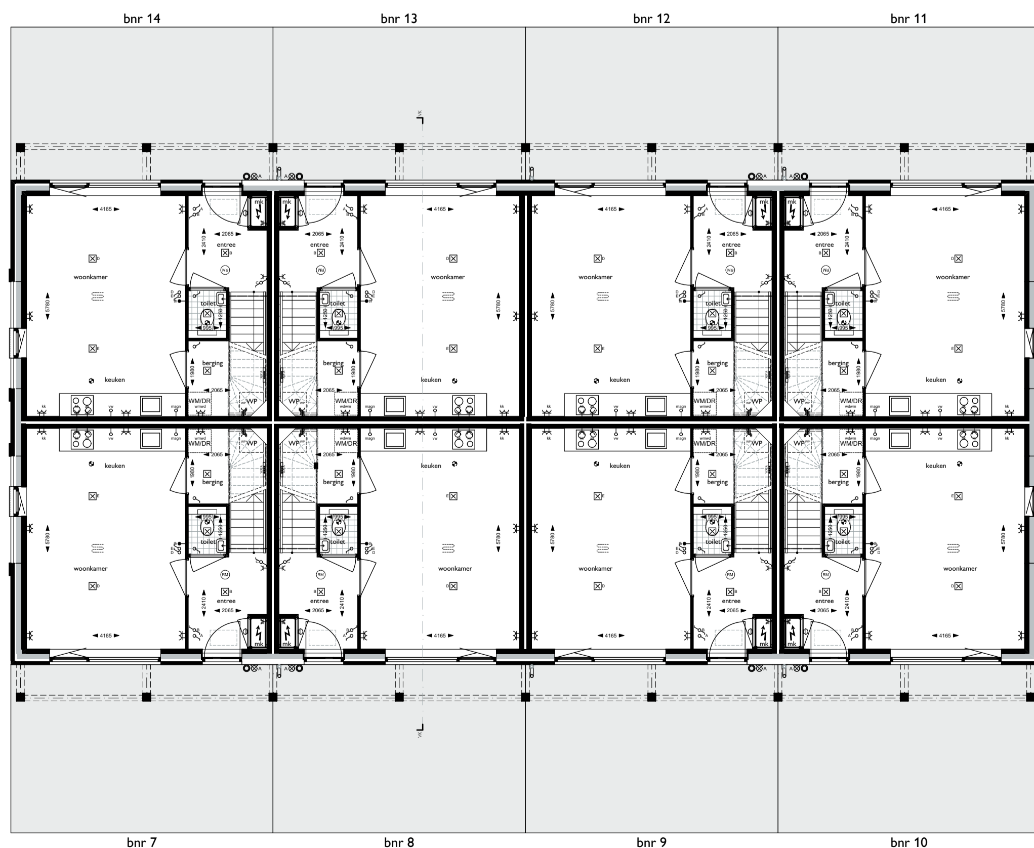
Begane grond
