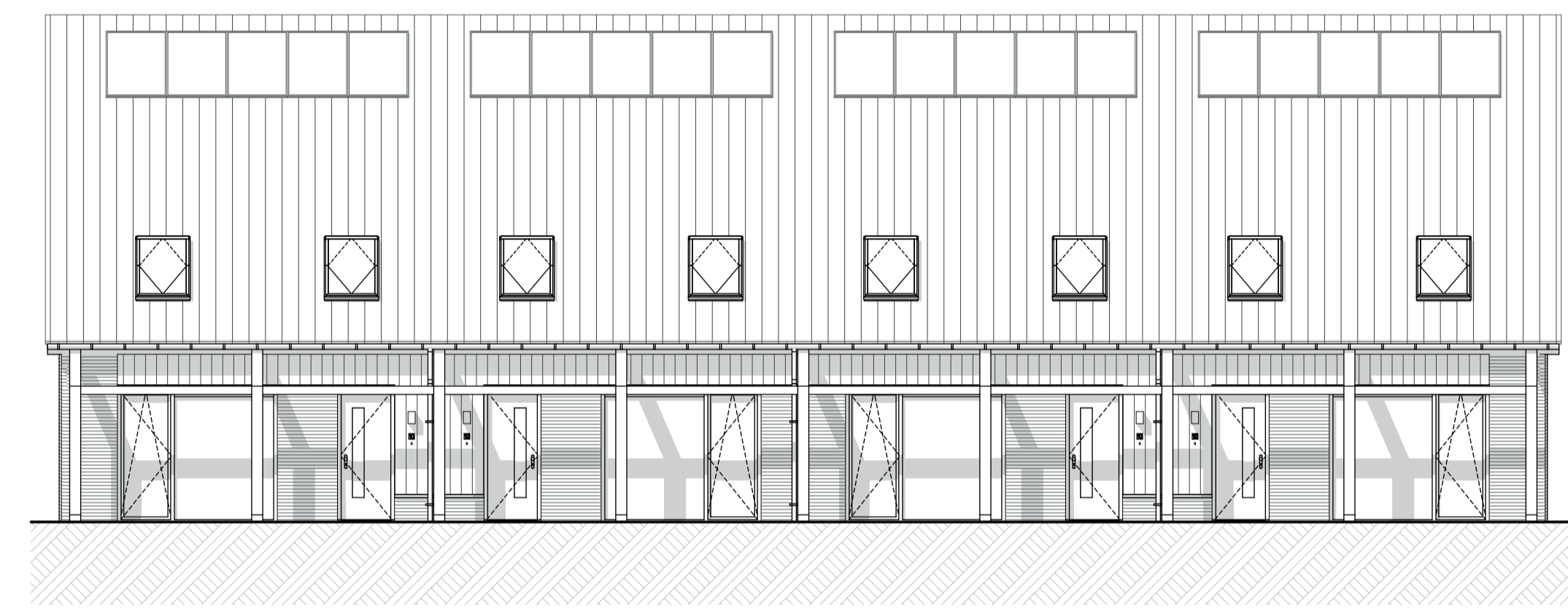
Achtergevel
