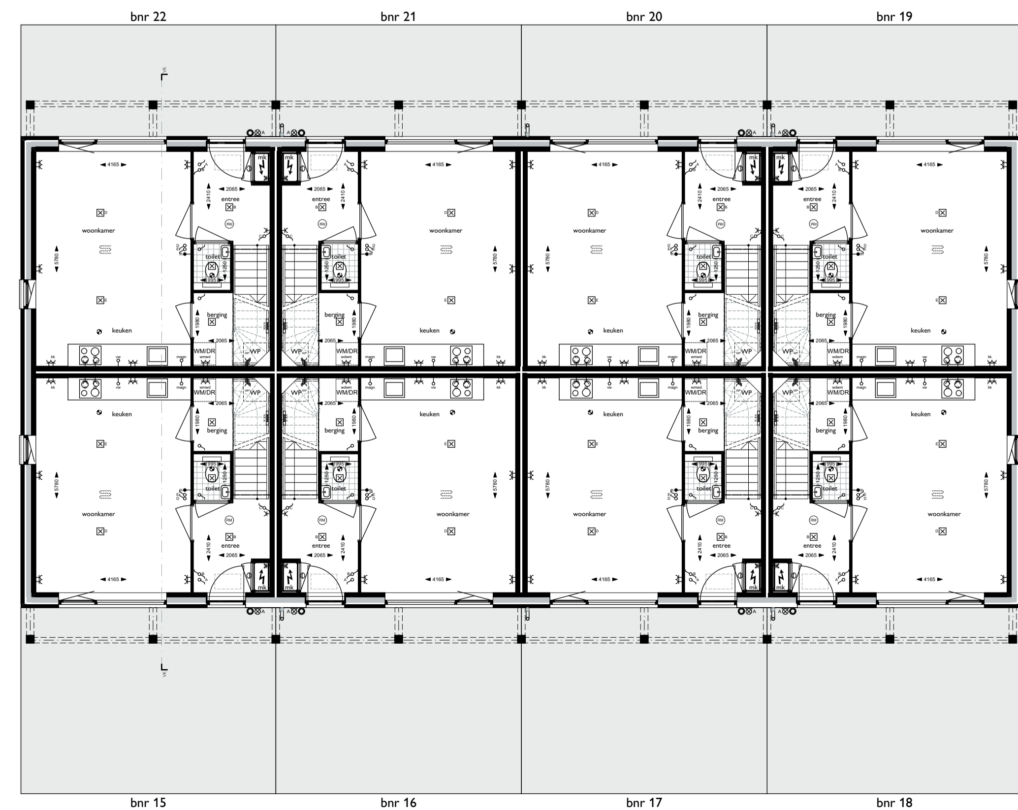
Begane grond
