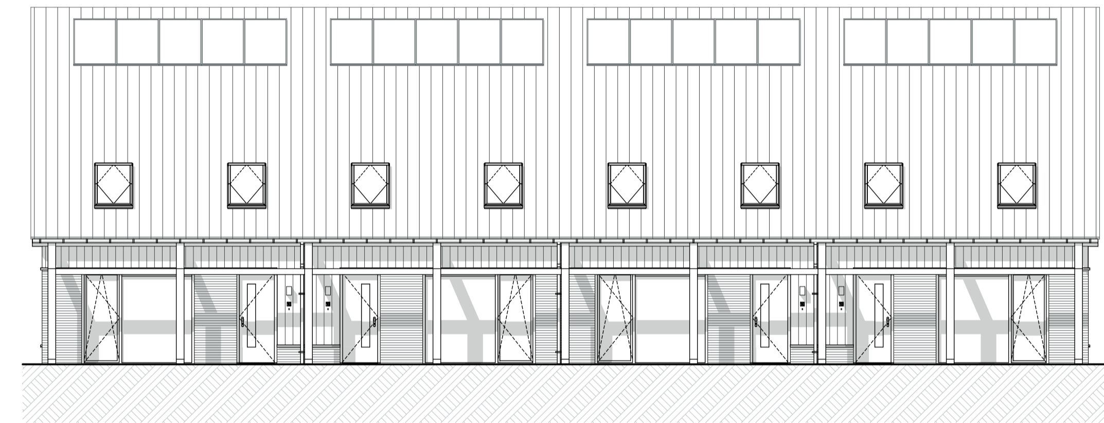
Achtergevel
