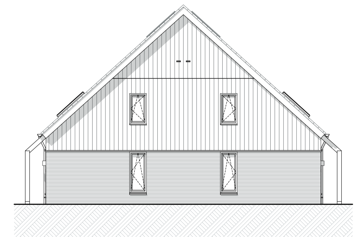
Rechtergevel
