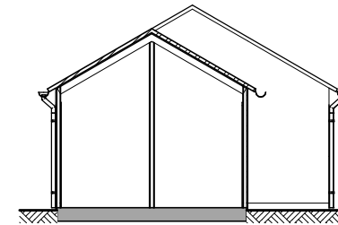
Doorsnede A-A
