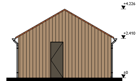
Rechtergevel
