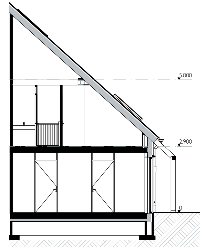
Doorsnede VK
