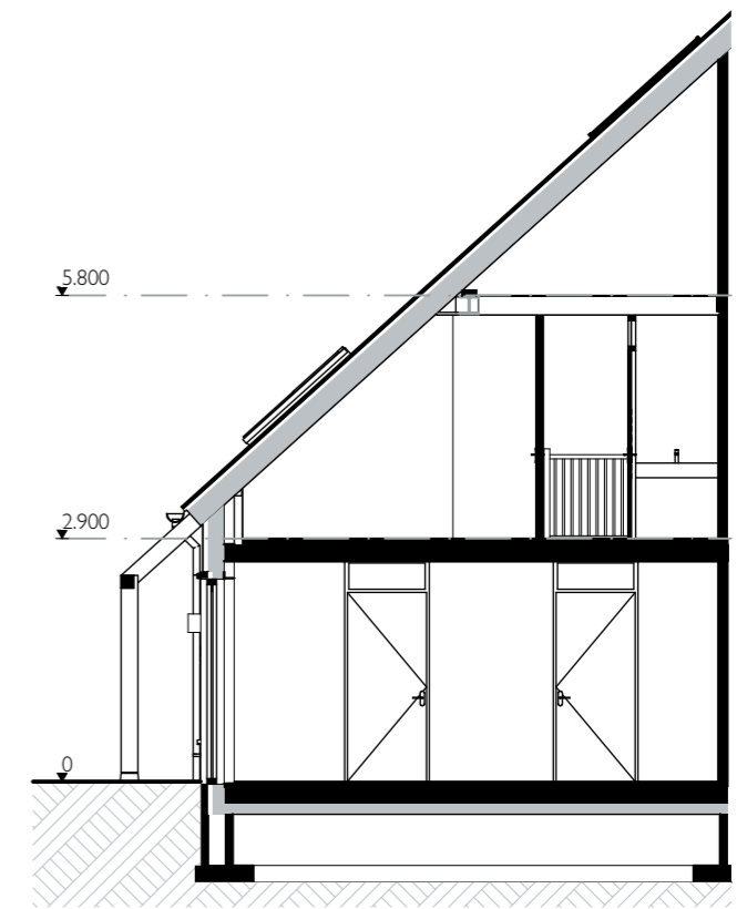
Doorsnede VK
