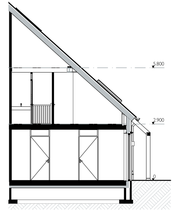
Doorsnede VK
